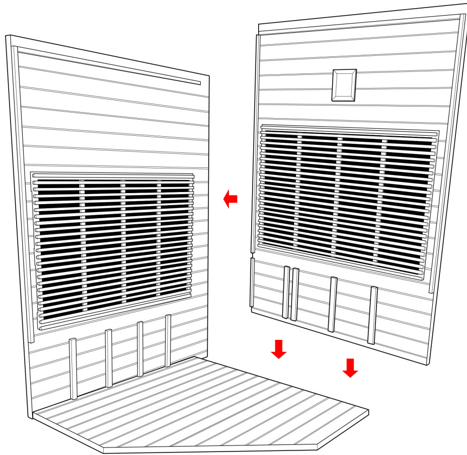
3x 35mm Screws
